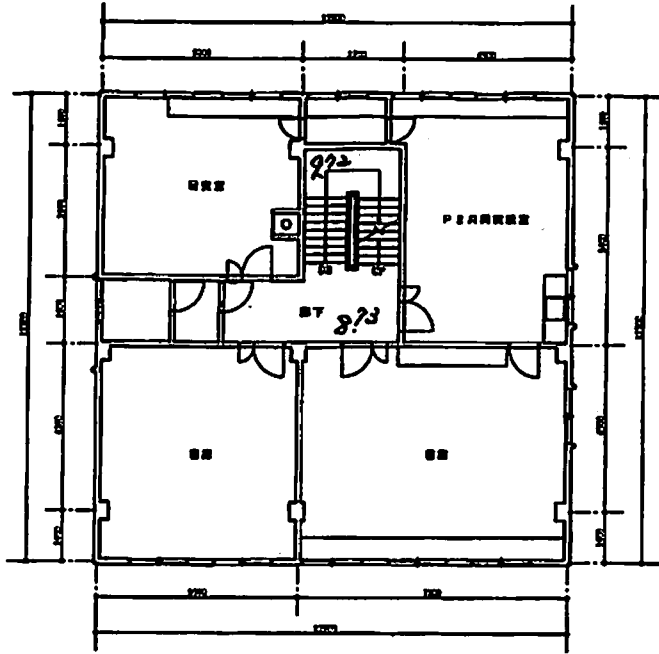
2階平面図
