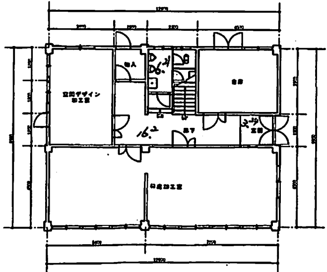
1階平面図
