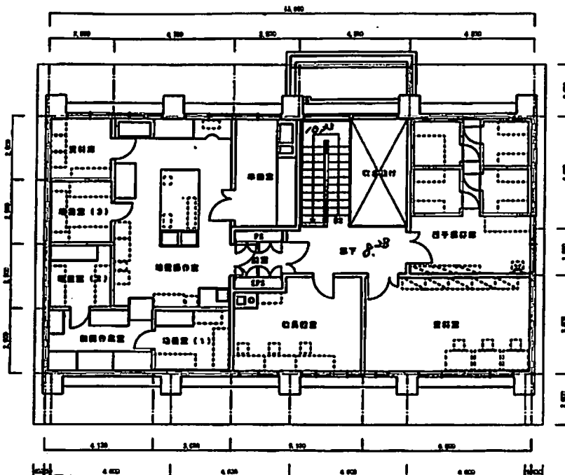
2階平面図
