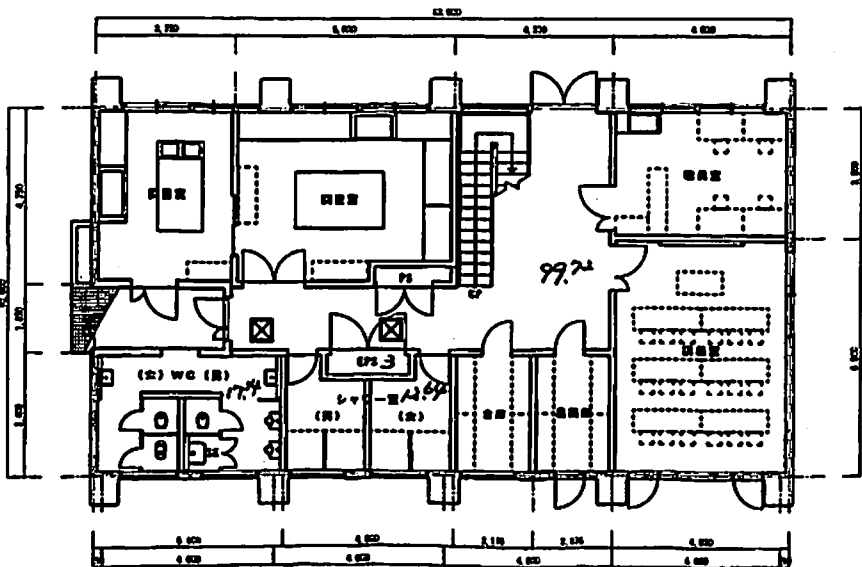
1階平面図
